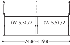
品名/OWR突張2375-120 S サイズ/W74.8~119.8×D17.5×H23cm 梱包サイズ/W134.7×D36×H7.3cm 重量/6.4~8.1kg
