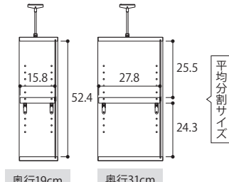
品名/OWR突張75675-120 R サイズ/W74.8~119.8×D29.5×H56.1cm 梱包サイズ/W130×D32.2×H12.5cm 重量/14.9~18.3kg
