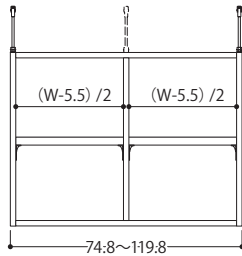
品名/OWR突張75675-120 S サイズ/W74.8~119.8×D17.5×H56.1cm 梱包サイズ/W134.7×D36×H7.3cm 重量/12~15kg
