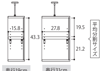
品名/OWR突張74775-120 R サイズ/W74.8~119.8×D29.5×H47cm 梱包サイズ/W130×D32.2×H12.5cm 重量/14~17.3kg
