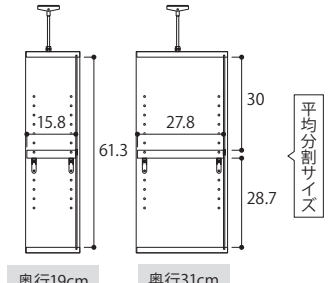
品名/OWR突張76575-120 R サイズ/W74.8~119.8×D29.5×H65cm 梱包サイズ/W130×D32.2×H12.5cm 重量/15.8~19.2kg
