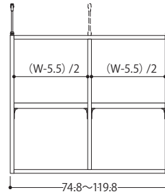
品名/OWR突張76575-120 S サイズ/W74.8~119.8×D17.5×H65cm 梱包サイズ/W134.7×D36×H7.3cm 重量/12.7~15.8kg
