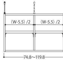
品名/OWR突張74775-120 S サイズ/W74.8~119.8×D17.5×H47cm 梱包サイズ/W134.7×D36×H7.3cm 重量/11.2~14.2kg
