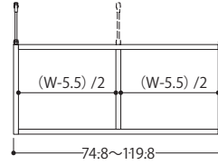
品名/OWR突張3275-120 S サイズ/W74.8~119.8×D17.5×H32cm 梱包サイズ/W134.7×D36×H7.3cm 重量/7.1~8.9kg
