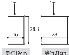
品名/OWR突張3275-120 R サイズ/W74.8~119.8×D29.5×H32cm 梱包サイズ/W130×D32.2×H12.5cm 重量/7.3~8.7kg
