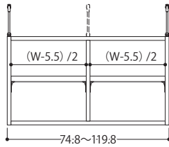
品名/OWR突張74175-120 S サイズ/W74.8~119.8×D17.5×H41cm 梱包サイズ/W134.7×D36×H7.3cm 重量/10.8~13.7kg
