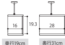
品名/OWR突張2375-120 R サイズ/W74.8~119.8×D29.5×H23cm 梱包サイズ/W130×D32.2×H12.5cm 重量/6.4~7.7kg
