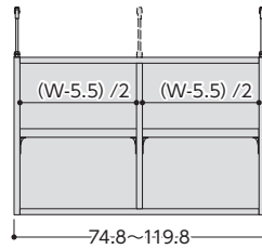
品名/OWR突張タフ4775-120 S サイズ/W74.8~119.8×D17.5×H47cm 梱包サイズ/W134.7×D36×H7.3cm 重量/11.2~14.2kg
