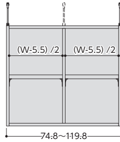
品名/OWR突張タフ6575-120 S サイズ/W74.8~119.8×D17.5×H65cm 梱包サイズ/W134.7×D36×H7.3cm 重量/12.7~15.8kg
