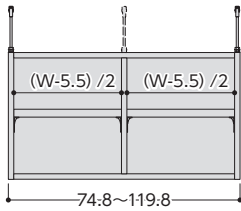
品名/OWR突張タフ4175-120 S サイズ/W74.8~119.8×D17.5×H41cm 梱包サイズ/W134.7×D36×H7.3cm 重量/10.8~13.7kg
