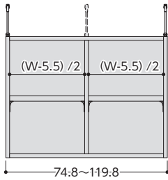
品名/OWR突張タフ5675-120 S サイズ/W74.8~119.8×D17.5×H56.1cm 梱包サイズ/W134.7×D36×H7.3cm 重量/12~15kg
